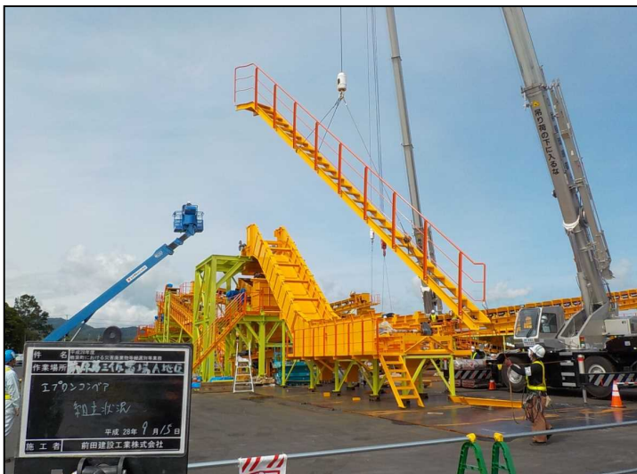
■エプロンコンベヤの組立状況 2016年9月15日 撮影
