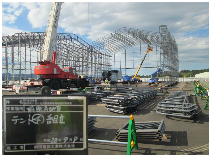
■仮設テントの設置状況 2016年9月9日 撮影
